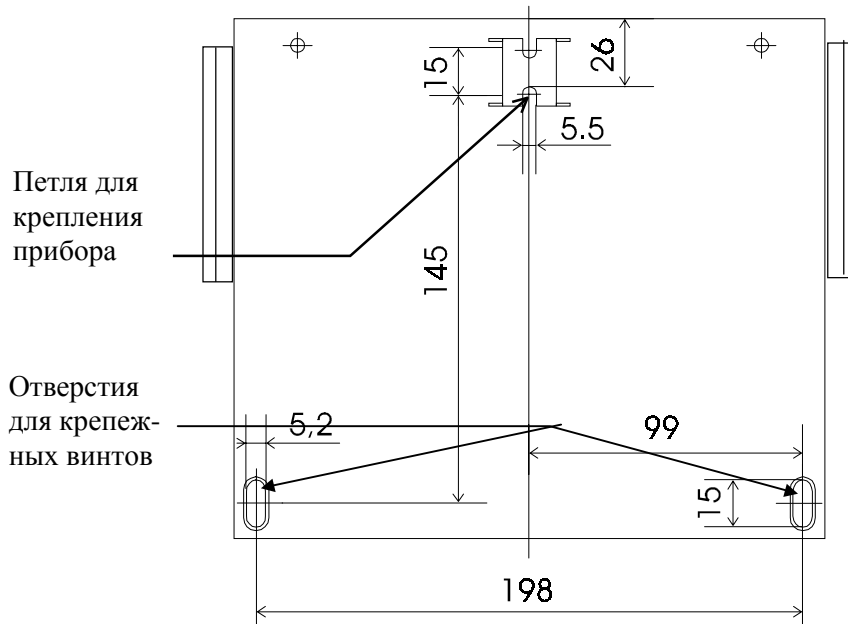
Рисунок 3.3 Сумматор СПЕ542. Вид сзади
