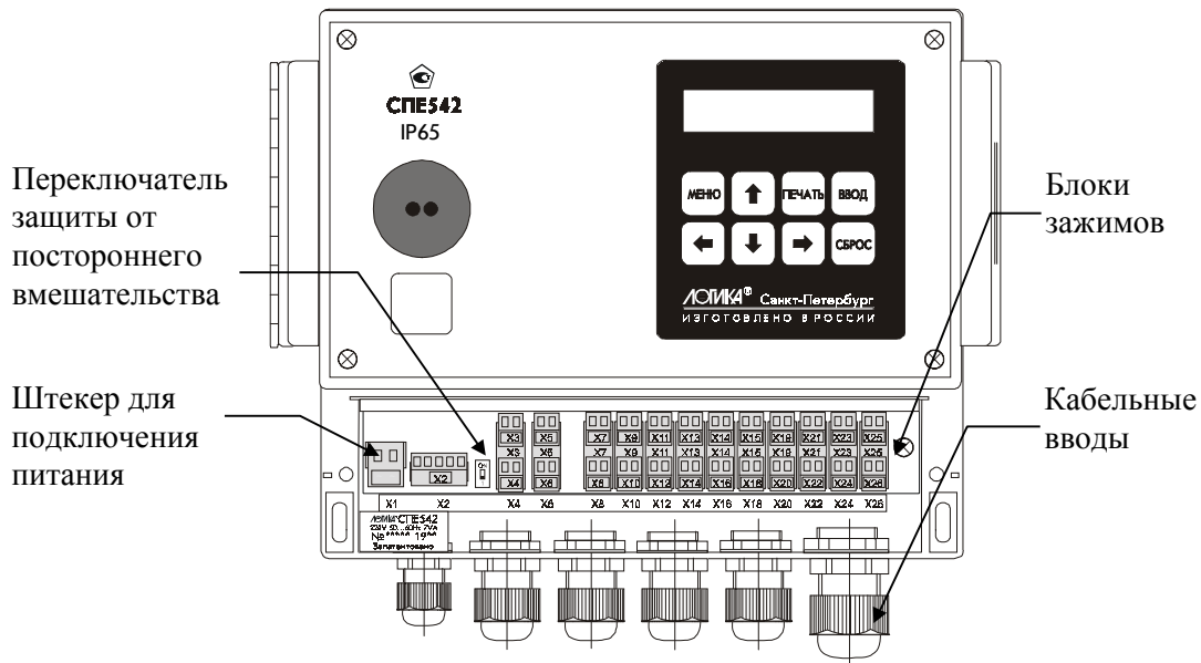
Рисунок 3.2 Сумматор СПЕ542. Вид спереди.
