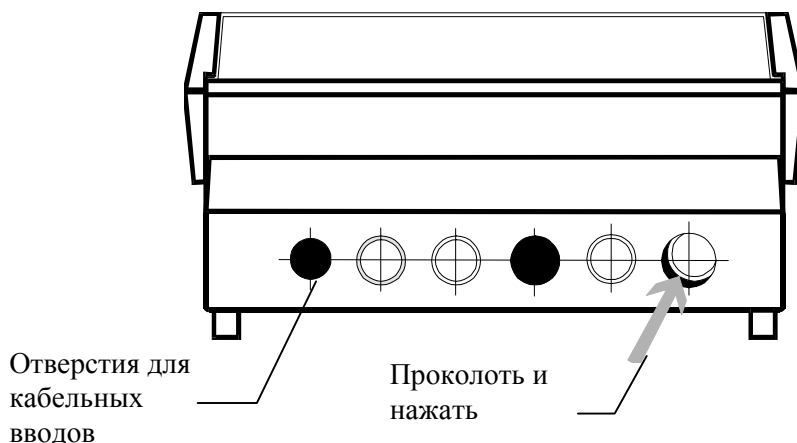
Рисунок 3.4 Сумматор СПЕ542. Вид снизу
