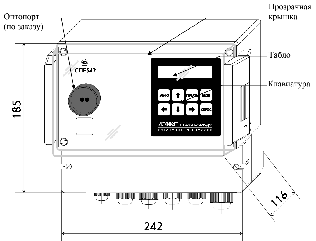
Рисунок 3.1 Внешний вид сумматора СПЕ542
