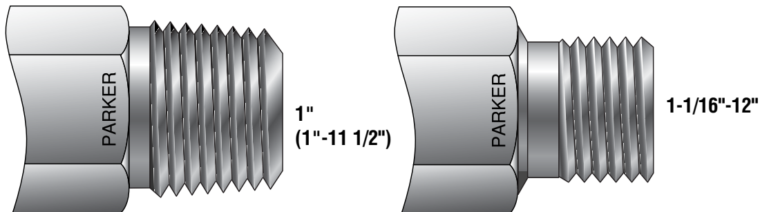
Стандарт США Резьба трубы (норм. трубная резьба)
