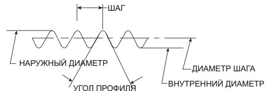
ТРУБОПРОВОДНАЯ РЕЗЬБА N.P.T.
