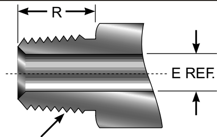
ТРУБОПРОВОДНАЯ РЕЗЬБА N.P.T.
